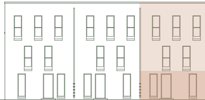
Frontansicht (Nord)
