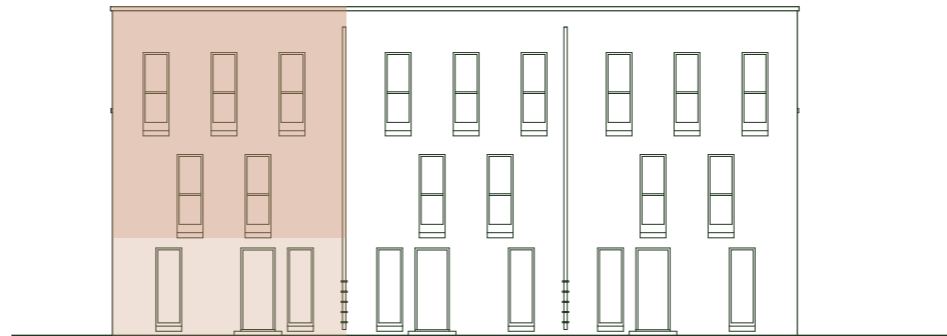
Frontansicht (Nord)
